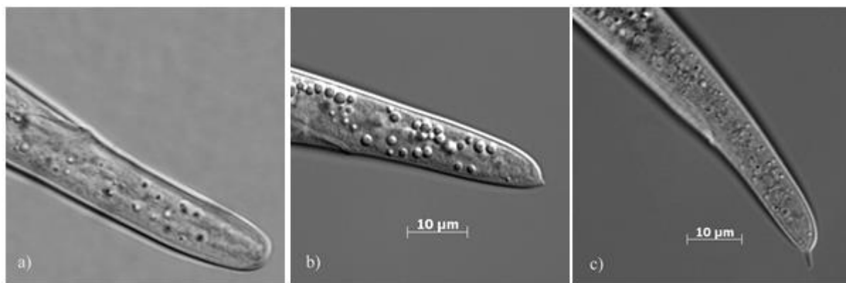
Рис. 4. Разновидности хвостов у самок Bursaphelenchus xylophilus : а) круглый (увеличение \times 1000 ); б) с небольшим выступом; и с) с мукро.
