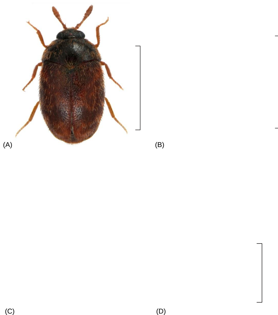
Рисунок 2: Trogoderma granarium : (A) имаго, самка; (B) сравнение формы самки (слева) и самца (справа); (C) молодая личинка; (D) зрелая личинка. Масштабная метка: (A), (B), (D) = 2 мм; (C) = 1 мм. ((A), Tomasz Klejdysz, Instytut Ochrony Roślin - Państwowy Instytut Badawczy, Poznań, Польша; (B), (D), Я.Б. Мордкович и Е.А. Соколов, ФГБУ "Всероссийский центр карантина растений", Быково, Россия) (C), Cornel Adler, Julius Kühn-Institut; (JKI) Германия)
