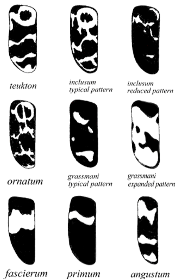
Рисунок 3: Рисунок светлых участков на надкрыльях видов Trogoderma (Beal, 1954)
